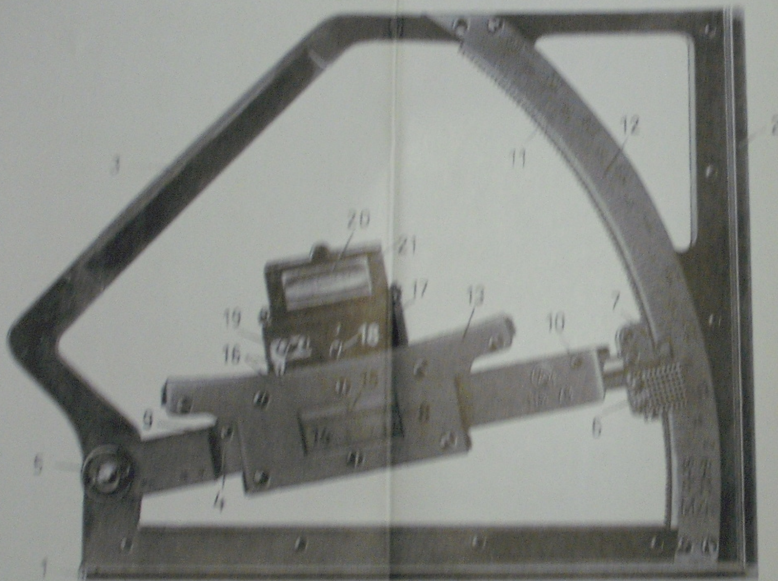
4 M. SZINTEZŐ NEGYEDLŐ bal oldalról.
