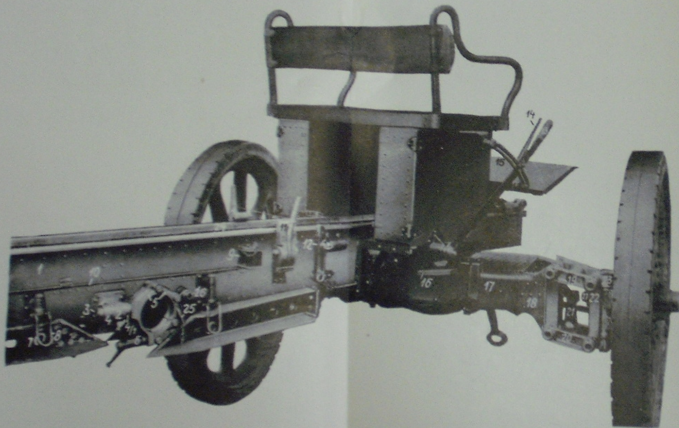
CSŐKOCSI (előlső része).
